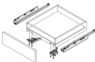
4-seitiger Schubkasten
