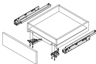
4-seitiger Schubkasten
