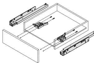
3-seitiger Schubkasten
