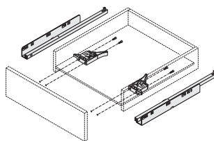
3-seitiger Schubkasten
