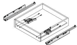
Innenschub
